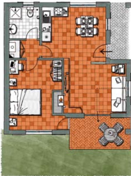
Voorbeeld: Woning A (begane grond)
